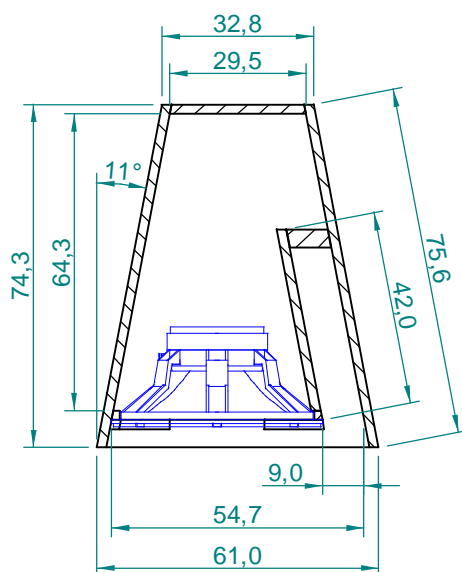
Corte B-B
