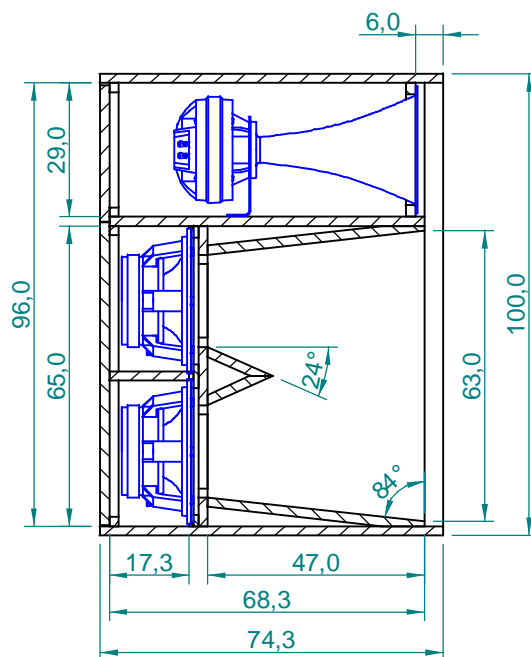
Corte A-A
