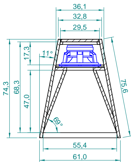
Corte B-B
